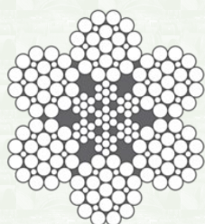
6x25F+IWRC
