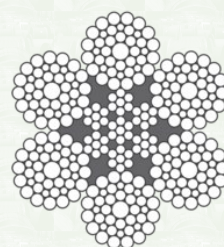
6x36WS+IWRC
